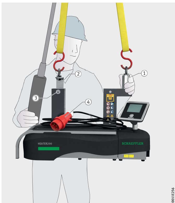
Рисунок 21 Перемещение HEATER200
