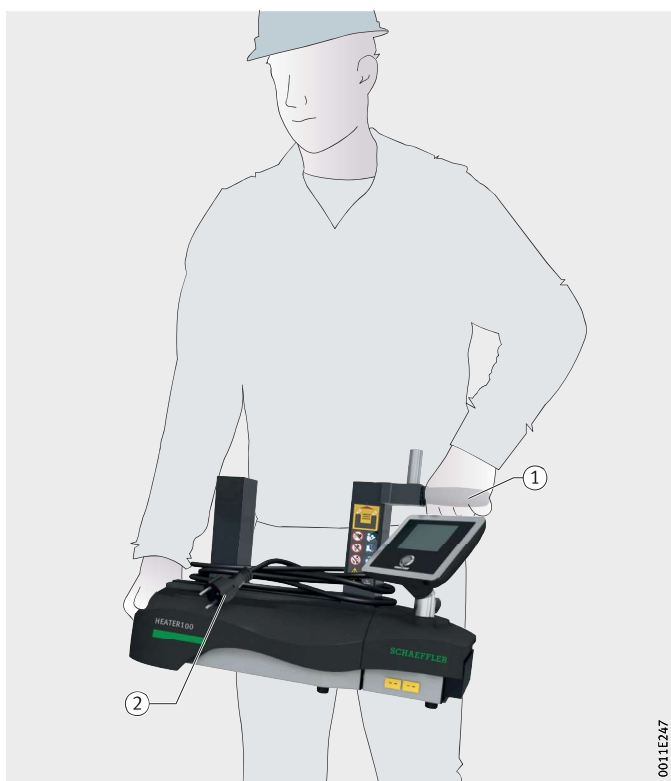
Рисунок 20 Перемещение HEATER100
