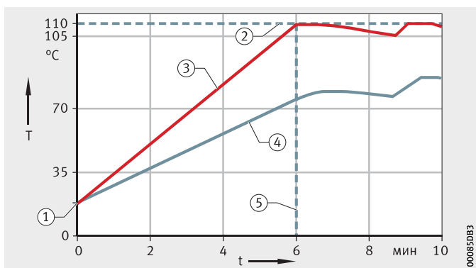
Рисунок 14 Управление по температуре
