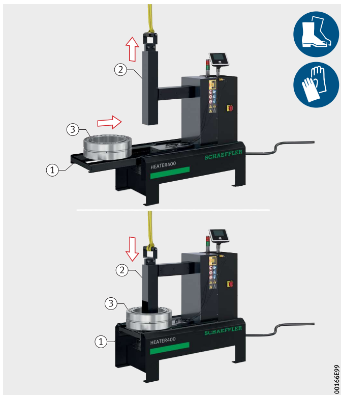
Рисунок 40 Выбор положения подшипника качения, вертикальная планка
