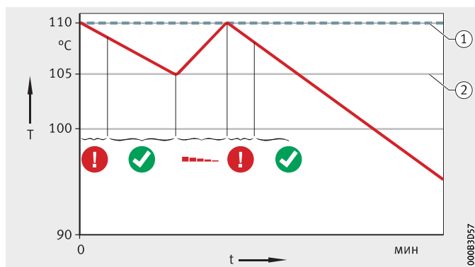
Рисунок 18 Конец поддержания температуры
