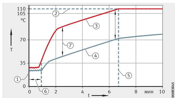
Рисунок 16 Управление Delta-T
