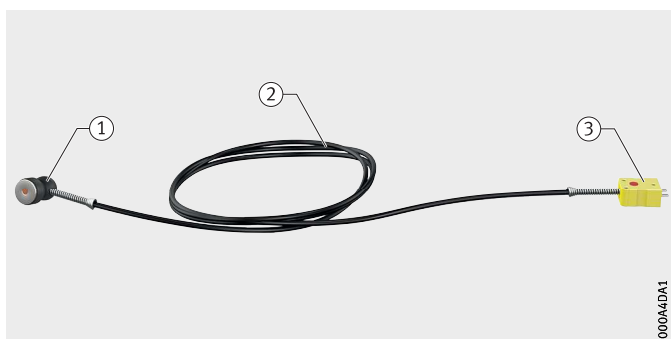
Рисунок 9 Датчик температуры
