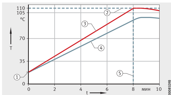
Рисунок 15 Управление по профилю изменения
