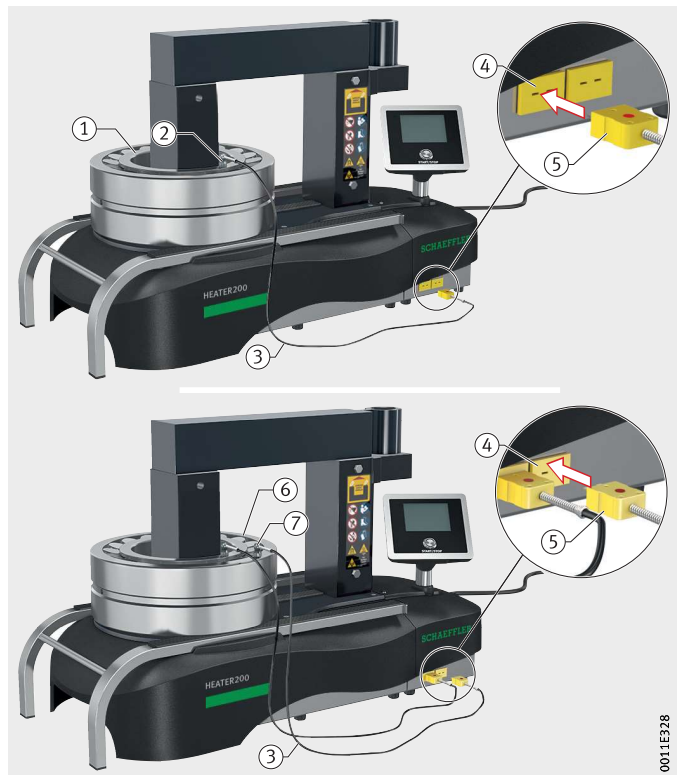
Рисунок 42 Подключение и настройка датчика температуры
