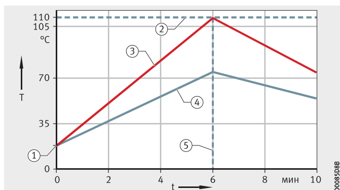
Рисунок 13 Управление по времени
