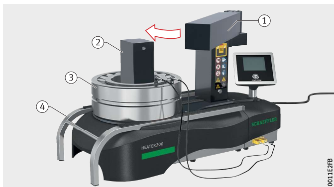
Рисунок 39 Подшипник качения, горизонтально уложенный, поворотная планка
