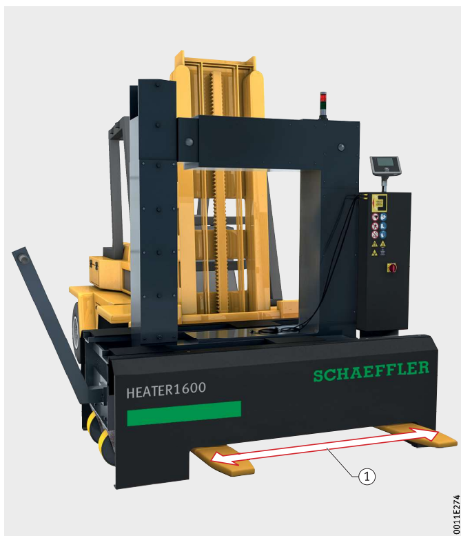
Рисунок 23 Перемещение HEATER1600
