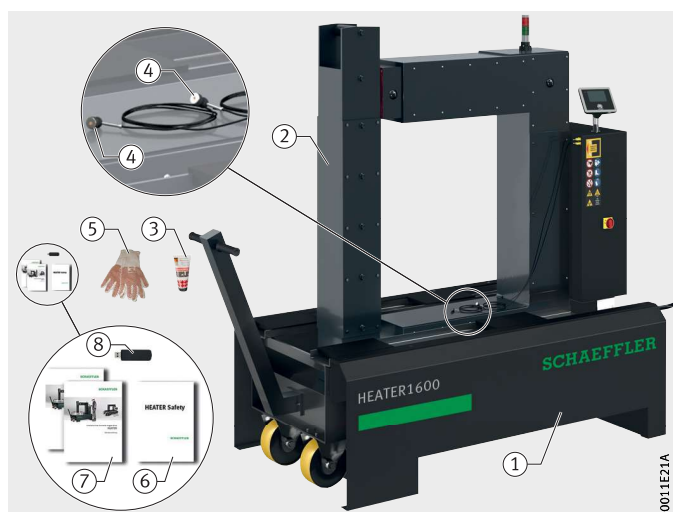
Рисунок 7 Комплект поставки нагревателя HEATER1600
