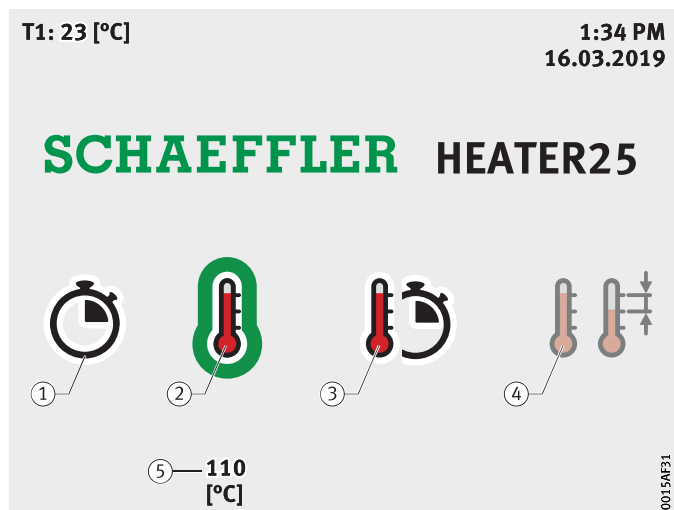
Рисунок 11 Методы нагрева, символы
