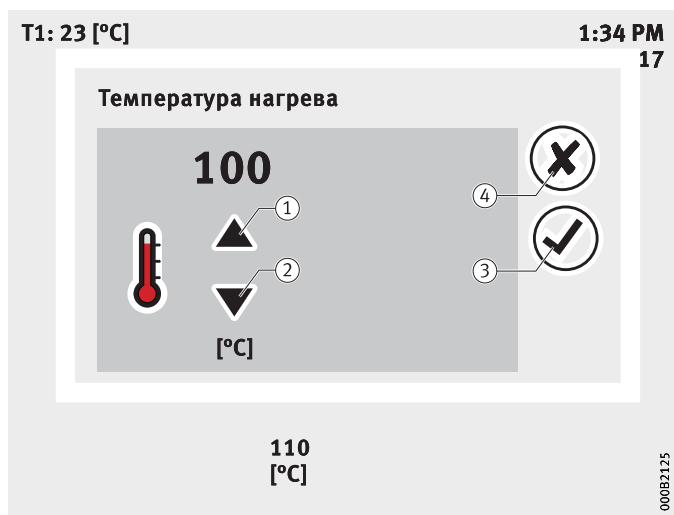
Рисунок 44 Окно температуры нагрева
