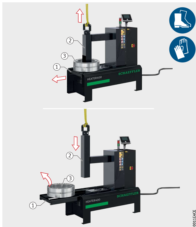
Рисунок 51 Снятие подшипника качения
