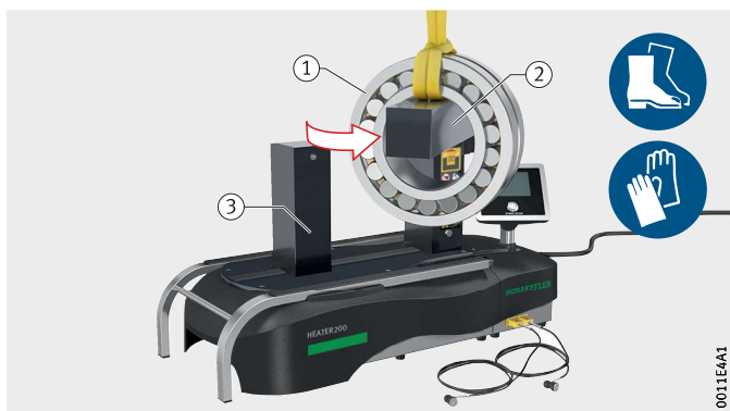
Рисунок 49 Снятие подвешенного подшипника качения с поворотной планки
