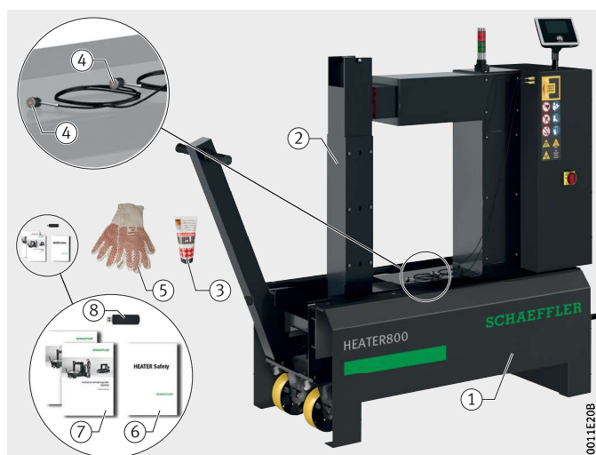
Рисунок 6 Комплект поставки нагревателя HEATER800
