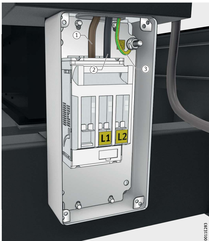
Рисунок 27 Сетевое подключение HEATER1600
