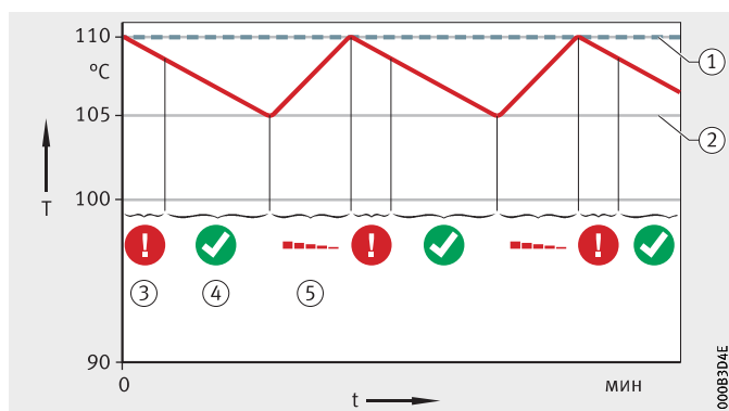
Рисунок 17 Охлаждение и нагрев
