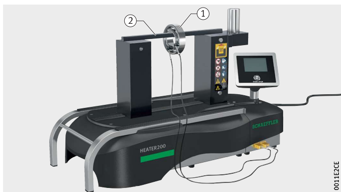
Рисунок 36 Подшипник качения, подвешенный, опорная планка
