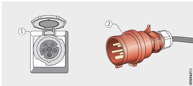
Рисунок 26 Электропитание HEATER200, HEATER400 и HEATER800
